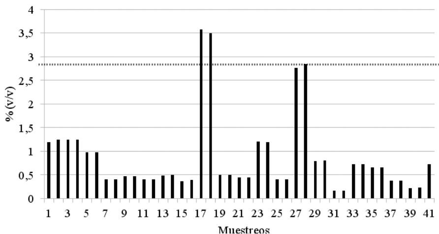
Figura 6: Niveles de benceno en nafta virgen. Corresponde a los resultados obtenidos de benceno en nafta virgen durante todo el mes de febrero 2017.
