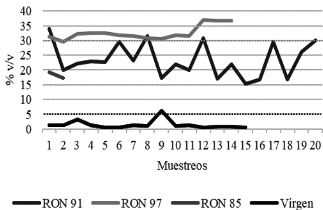
Figura 1: Fracción de hidrocarburos aromáticos en gasolinas del tipo RON 97, RON 91, RON 85 y Nafta virgen. Corresponde al período comprendido entre abril y agosto 2017.
