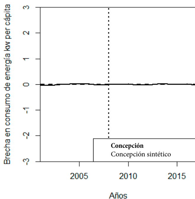
Figura 40: Brecha entre Concepción y Concepción sintético
